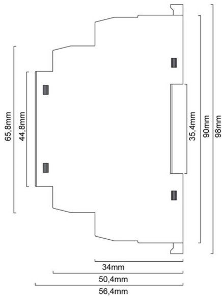
Geometrie Hutschienenmodul
