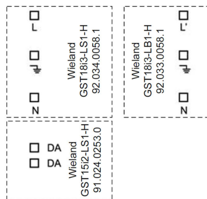
Anschlussplan RM16-CEL
