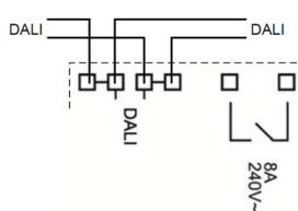
Anschlussplan RM8
