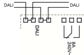
Anschlussplan RM16
