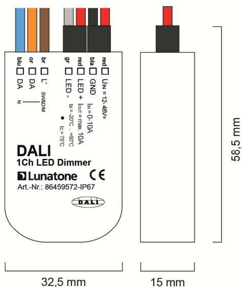
Abmessungen
