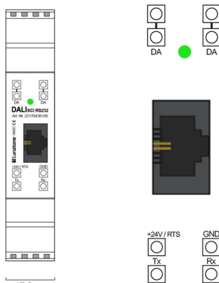
Anschlussbelegung DALI SCI RS232
